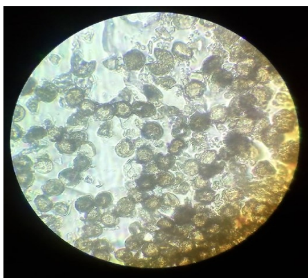
Споры твёрдой головни пшеницы ( Tilletia levis , T. caries , T. intermedia )
